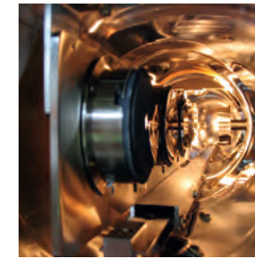
Blick ins Vakuum einer Epitaxie-Anlage, Gruppe Prof. Bougeard.
